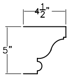
EDGE DETAIL
