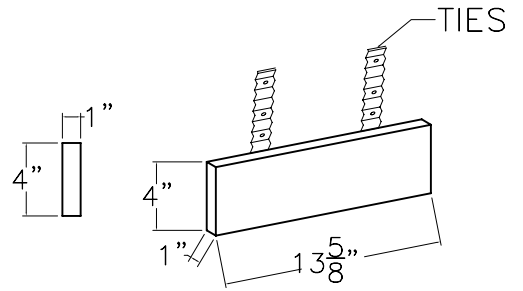
EF-414 EDGE FACING
